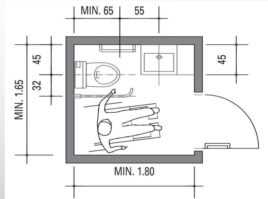
Plan de cotes - Vue du dessus des WC pour PMR
