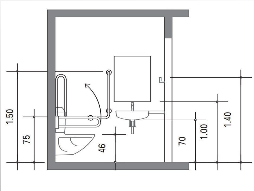
Plan de cotes - Vue latérale des WC pour PMR
